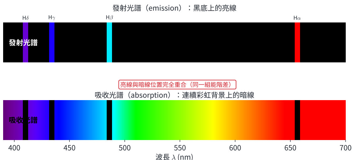
圖 6-5：發射光譜與吸收光譜對照（以氫原子巴耳末系 H\alpha 、 H\beta 、 H\gamma 、 H\delta 為例）。上——發射光譜為黑底上的幾條亮線；下——吸收光譜為連續彩虹背景上的幾條暗線。同一元素的亮線與暗線位置完全重合，因為兩者來自同一組能階差。
